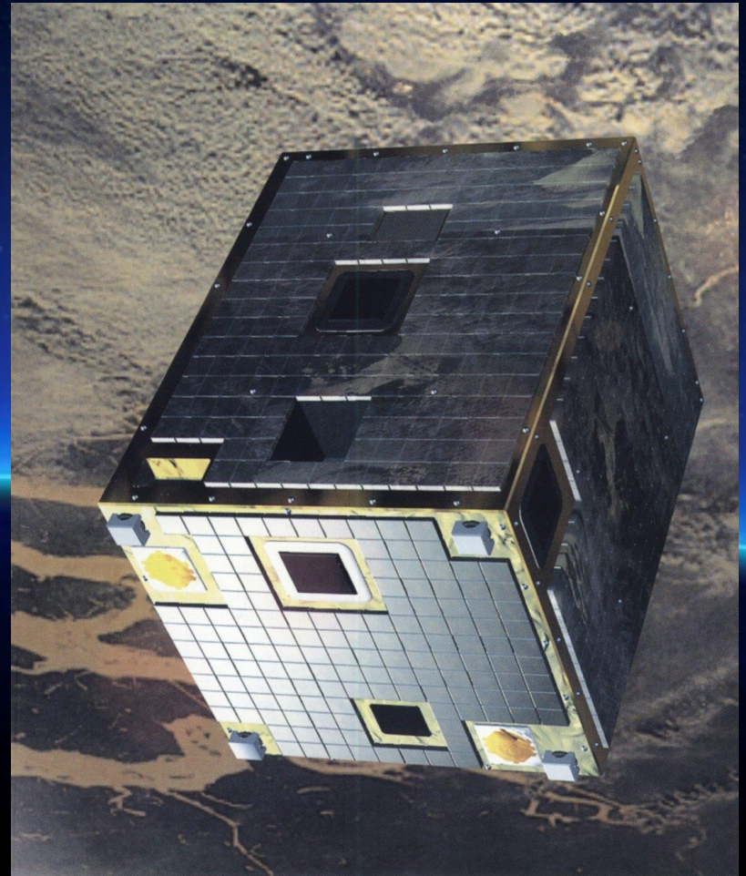
Υπερφασματικός CHRIS-PROBA
