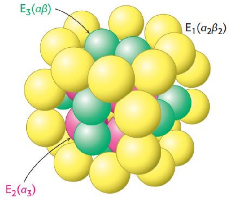
ΕΙΚΟΝΑ 17.7 Σχηματική αναπαράσταση του συμπλέγματος της πυροσταφυλικής αφυδρογονάσης. Ο πυρήνας της τρανσακετυλάσης ( E_2 ) φαίνεται με κόκκινο, η συνιστώσα της πυροσταφυλικής αφυδρογονάσης ( E_1 ) με κίτρινο και η διυδρολιποϋλο-αφυδρογονάση ( E_3 ) με πράσινο.
