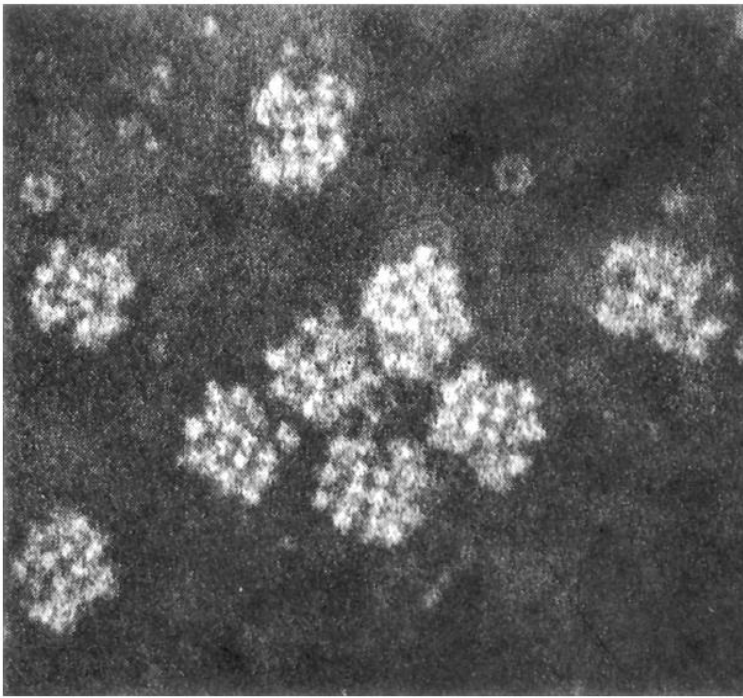
Εικόνα 17.5 Ηλεκτρονιομικρογραφία του συμπλέγματος της πυροσταφυλικής αφυδρογονάσης από την E. coli . [Ευγενική προσφορά Dr. Lester Reed.]
