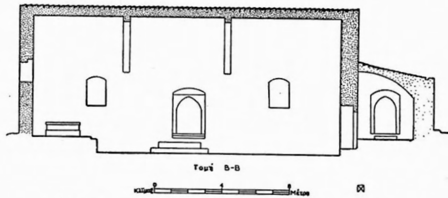
Εικ. 2. Τομή κατά μήκος του νοτίου κλίτους του ναού 'Αγ. Σπυρίδωνος.
