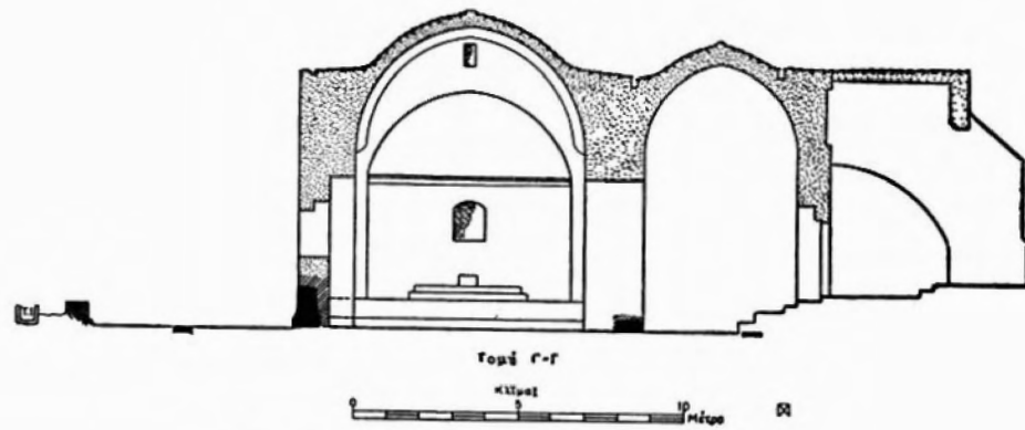
Εικ. 1. Τομή κατά πλάτος του ναού 'Αγ. Σπυρίδωνος.
