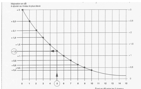
Fig. A.2 - « Addition » de deux niveaux sonores.
