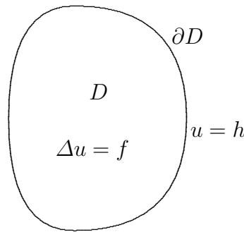
Σχήμα 6.1: Το πρόβλημα για την εξίσωση του Poisson με συνοριακές συνθήκες Dirichlet.
