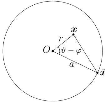
Σχήμα 6.3: Το πρόβλημα για την εξίσωση του Poisson στον κύκλο με συνοριακές συνθήκες Dirichlet.
