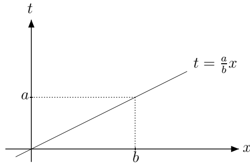
Σχήμα 1.1: Οι χαρακτηριστικές γραμμές της (1.10) έχουν εξισώσεις ax - bt = \text{σταθερά} , και είναι παράλληλες προς την ευθεία που διέρχεται από την αρχή των αξόνων και το σημείο (b, a) .
