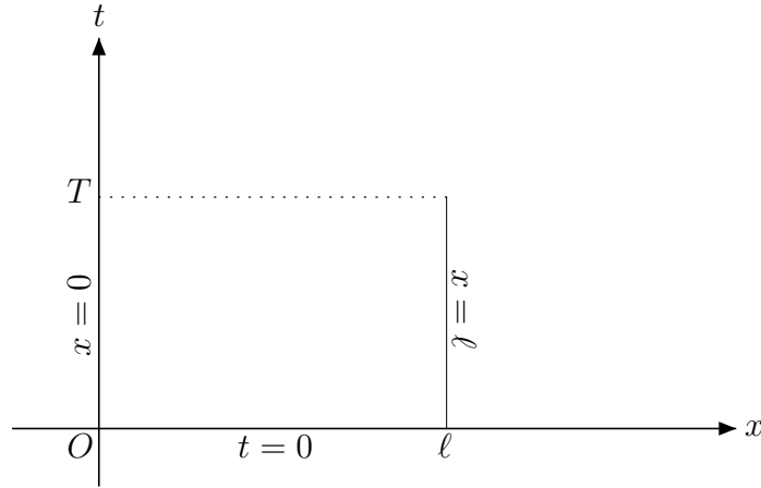
Σχήμα 3.1: Λύσεις της εξίσωσης της θερμότητας λαμβάνουν το μέγιστό τους στο ορθογώνιο [0, \ell] \times [0, T] και σε μια από τις τρεις πλευρές του που σχεδιάστηκαν με συνεχή γραμμή.
