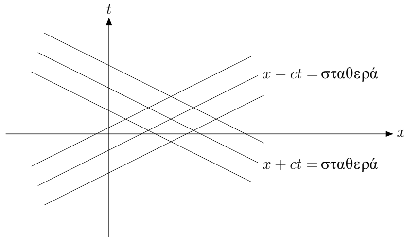
Σχήμα 2.1: Οικογένειες χαρακτηριστικών γραμμών για την κυματική εξίσωση.
