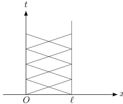
Σχήμα 2.10: Στα τρίγωνα και τους ρόμβους του σχήματος, που σχηματίζονται από το σύνορο και τις χαρακτηριστικές γραμμές, διαφορετικοί τύποι μας δίνουν τη λύση του προβλήματος (2.17).
