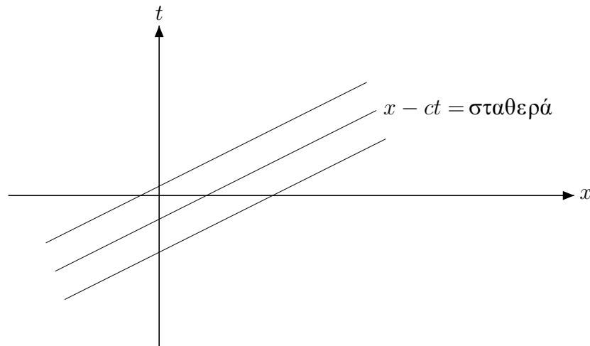
Σχήμα 1.3: Οικογένεια χαρακτηριστικών γραμμών της εξίσωσης μεταφοράς.
