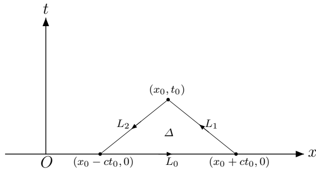
Σχήμα 2.13: Χαρακτηριστικό τρίγωνο του σημείου (x_0, t_0) .
