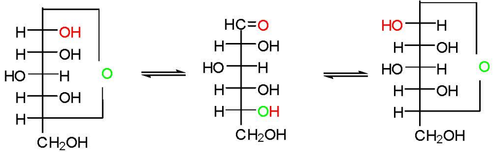
α-D-γλυκόπυρανόζη (36%)
