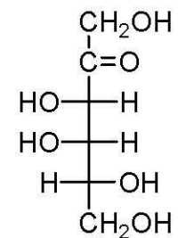
D-ταγκατόζη
