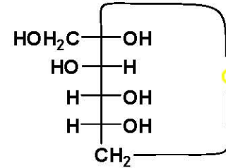
α-D-φρουκτοπιρανόζη
