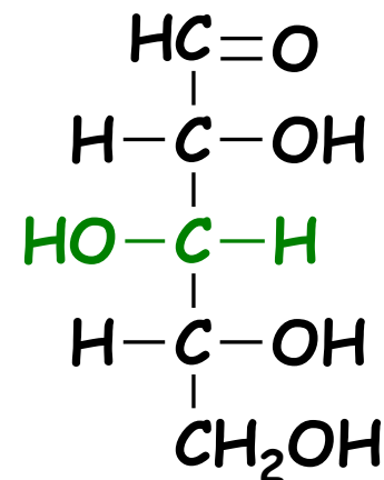
D-ξυλόζη
