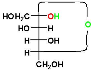
α-D-φρουκτοφουρανόζη
