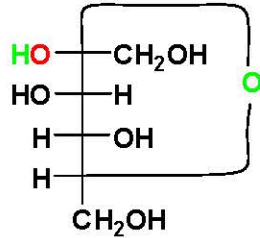
β-D-φρουκτοφουρανόζη
