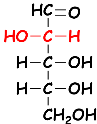
D-αραβινόζη
