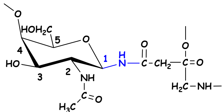
N-γλυκοζιτικός δεσμός
