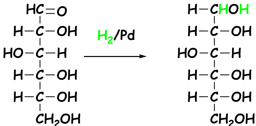
D-γλυκόζη
