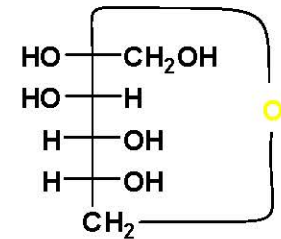
β-D-φρουκτοπιρανόζη
