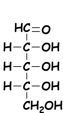
D-ριβόζη
