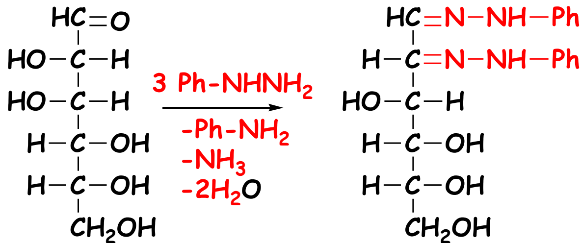
D-μανόζη
