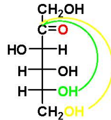
D-φρουκτόζη
