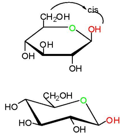
β-D-γλυκόπυρανόζη (64%)
