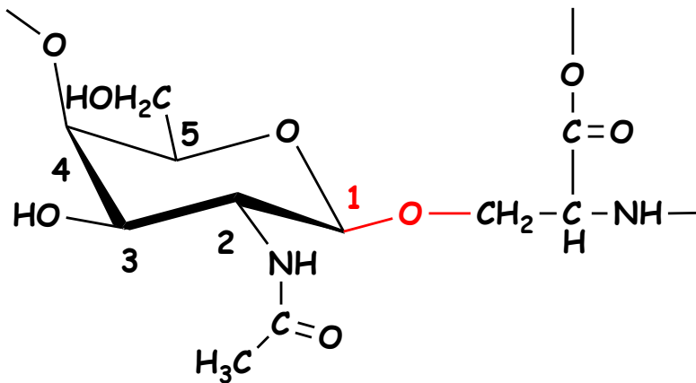
O-γλυκοζιτικός δεσμός
