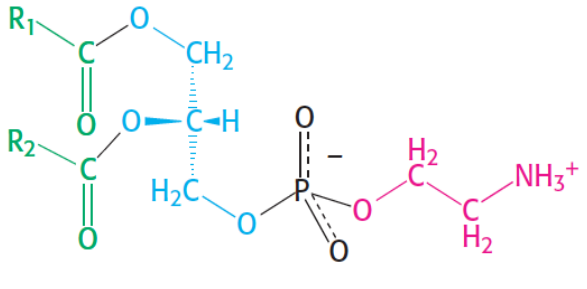
Φωσφατιδυλαιθανολαμίνη
