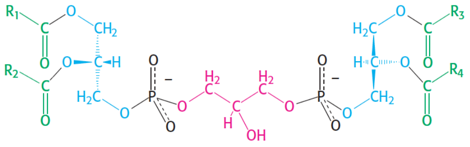
Διφωσφατιδυλογλυκερόλη (καρδιολιπίνη)
