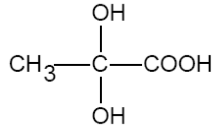
Γλυκερινικό οξύ
