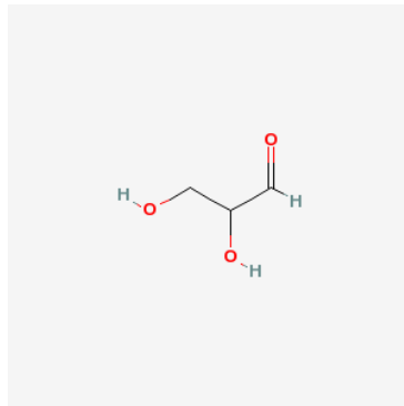
Γλυκεριναλδεύδη
