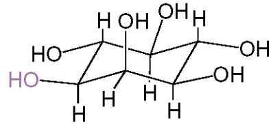
Ινοσιτόλη
