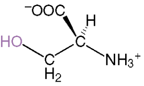
Σερίνη
