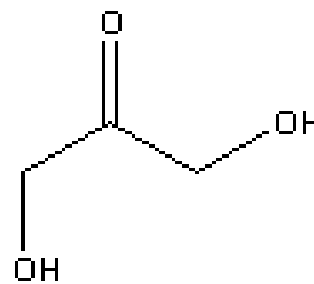
Διυδροξυπροπανόνη
