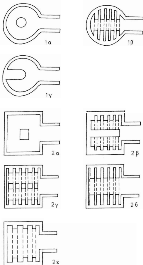
Εικ. 3. Τύποι διώροφων κλιβάνων ανοδικής καύσης.
