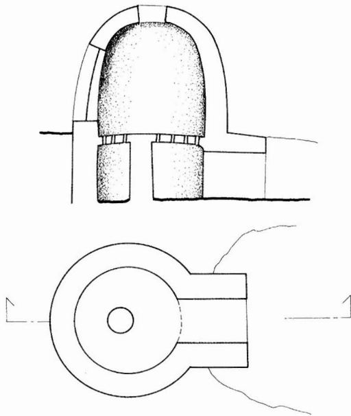
Εικ. 2. Διώροφος κλιβανος ανοδικής καύσης εργαστηρίου κεραμικής.
