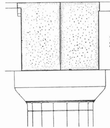
Εἰκ. 84. Τὸ ἐκ δύο κατὰ τὸ πάχος τεμαχίων ἐπιστύλιον τοῦ ἐν Σούνιῳ ναοῦ τοῦ Ποσειδῶνος. (Ὁρλάνδος)
