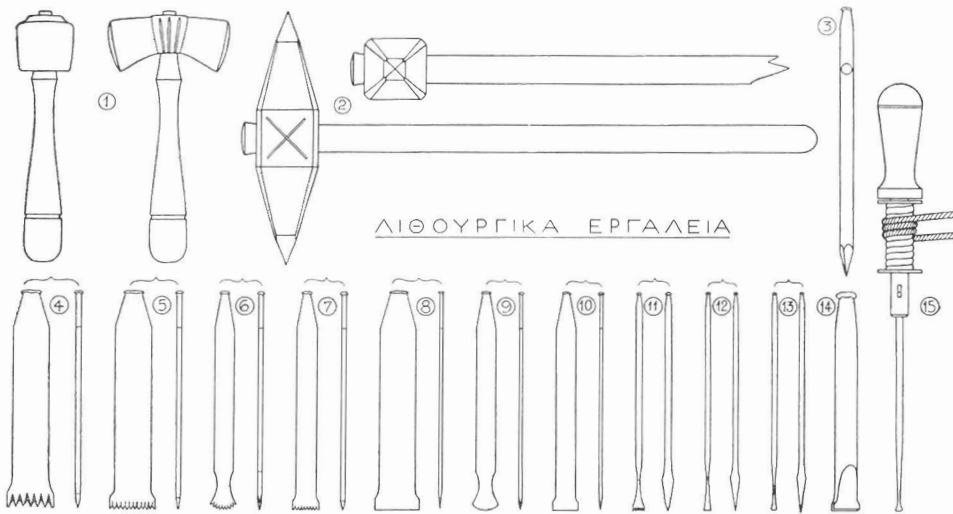
Εἰκ. 56. Σύγχρονα λιθουργικὰ ἐργαλεῖα: 1 μαντρακὸς 2 πικούνι 3 βελόνι 4 φαγάνα 5 ντισιλίδικο 6 λουκλούδικο ντισιλίδικο (διὰ κοιλότητος) 7 ντισιλιδάκι 8 λάμα 9 λαμάκι λουκλούδικο (διὰ γλυφῆς) 10 λαμάκι 11 καὶ 12 γλῶσσα 13 ποντίλι 14 κοπίδι 15 ἀρίδα.
