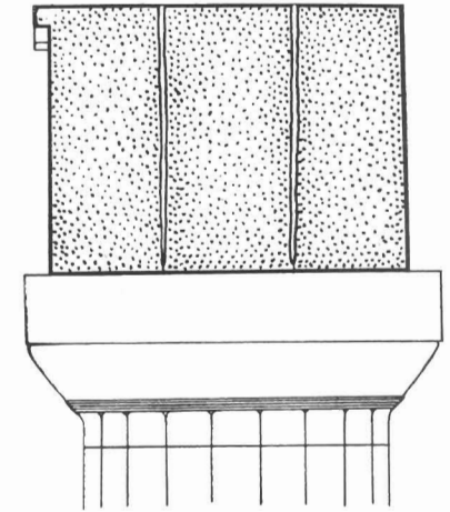
Εἰκ. 85. Τὸ ἐκ τριῶν κατὰ τὸ πάχος τεμαχίων ἐπιστύλιον τοῦ Παρθενῶνος. (Ὁρλάνδος)
