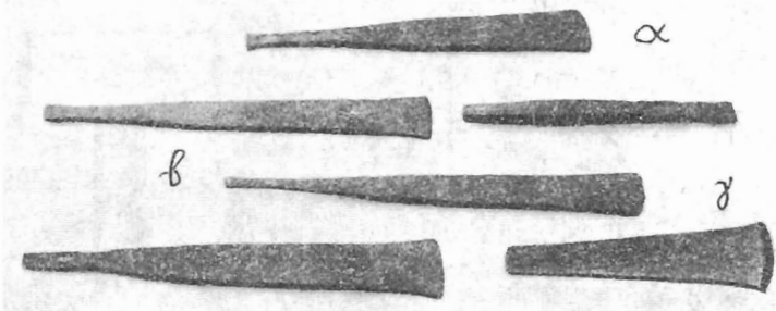
Εικ. 62. α, β Λιθουργικά έργαλεία (λείστρια) τής ΥΜ Ι περιόδου έκ Γουρνιών Κρήτης. Τό γ λείστριον (λάμα) τής χαλκής έποχής έκ Νισούρου (Walters).
