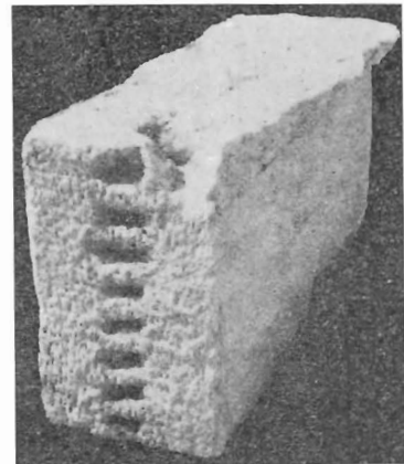
Εἰκ. 71. Διαδοχικὰ ἐπάλληλα μοχλοβόθρια ἐπὶ μεταδοκίῳ πλακῶς τοῦ Παρθενῶος.
