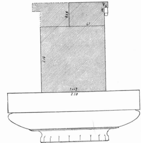
Εἰκ. 86. Τὸ ἐξ ἐνὸς κατὰ τὸ πάχος τεμαχίου ἐπιστύλιον τοῦ ἀρχαίου ναοῦ G τοῦ Σελινοῦντος. (Koldewey)
