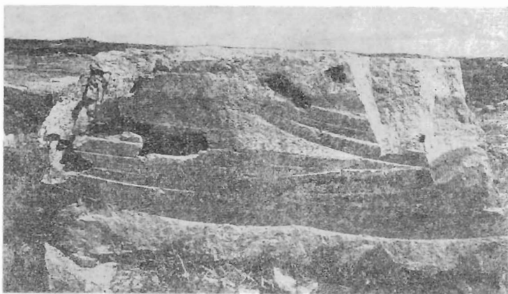
Εἰκ. 68. Ἰχνη τοῦ λιθοπρίονος ἐπὶ τῆς δυτικῆς παραστάδος τοῦ μεγάλου προπύλου τοῦ ἀνακτόρου τῆς Τίρυνθος (K. Müller).
