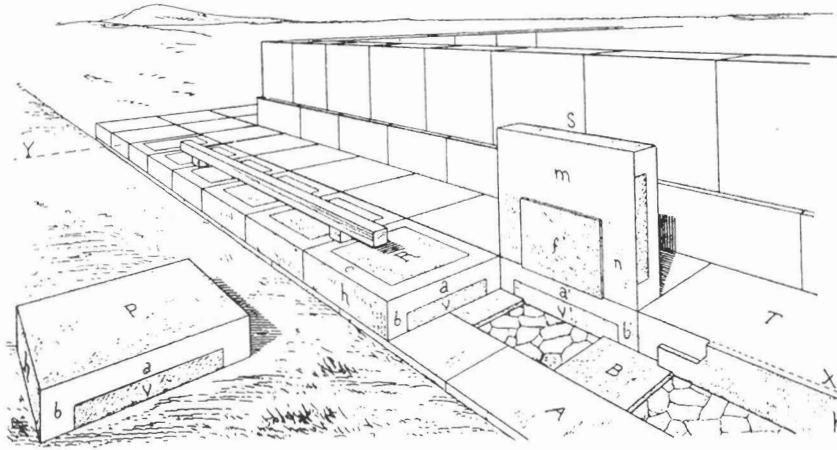
Εἰκ. 82. Ἀναπαράσταση ξυλίνου κανόνος βαίνοντος ἐπὶ κύβων στηριζομένου ἐπὶ τῆς περιτελείας τῶν καταστρωτῶρων τοῦ παρὰ τὴν Λεβάδειαν ναοῦ τοῦ βασιλέως Διός (Choisy).
