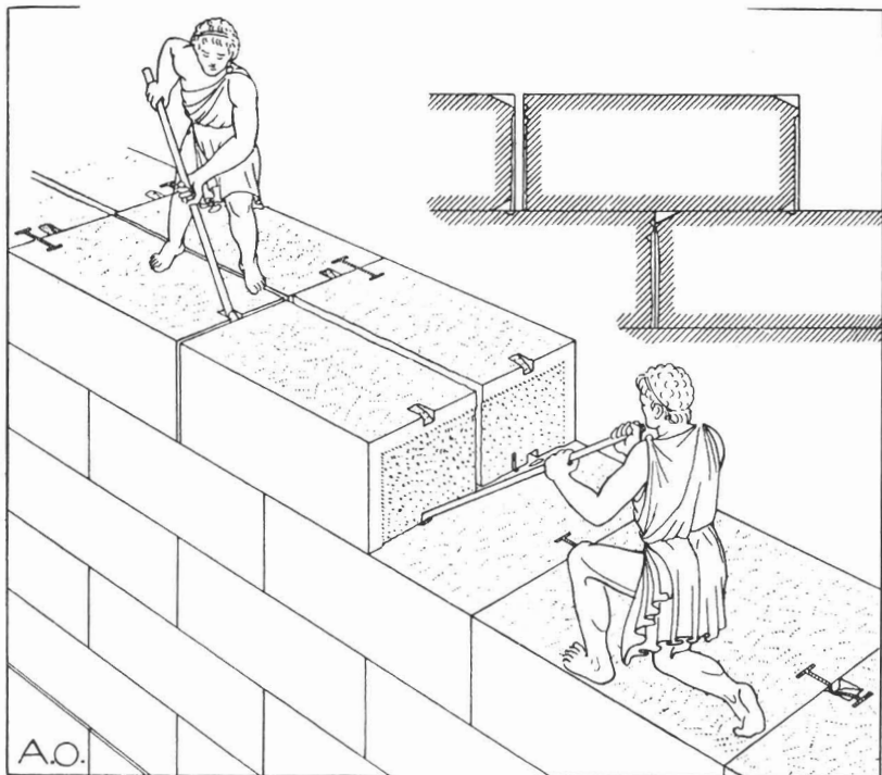
Εἰκ. 70. Χρήσις σιδηρῶν μοχλῶν πρὸς μετακίνησην τῶν λίθων τῆ βοηθείᾳ καὶ λοξῶν ἔγκοπῶν ἀνοιγομένων εἰς τὰς ἄνω καὶ τὰς κάτω κόψεις τῶν λίθων ('Ορλάνδος).
