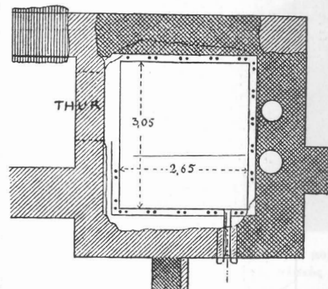
Εἰκ. 69. Κάτοψις τοῦ λουτροῦ τοῦ ἀνακτόρου τῆς Τίρυνθος ἐμφαίνουσα τὰς ἐπὶ τοῦ λίθου κυκλικὰς ὀπὰς (Dörpfeld).
