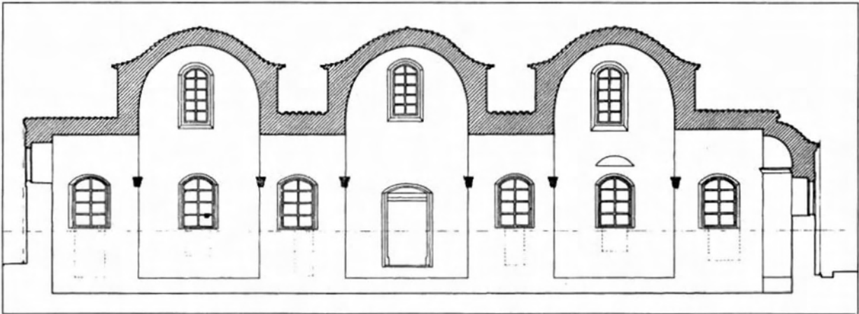
Σχ. 11. Τομή Γ-Γ'.
