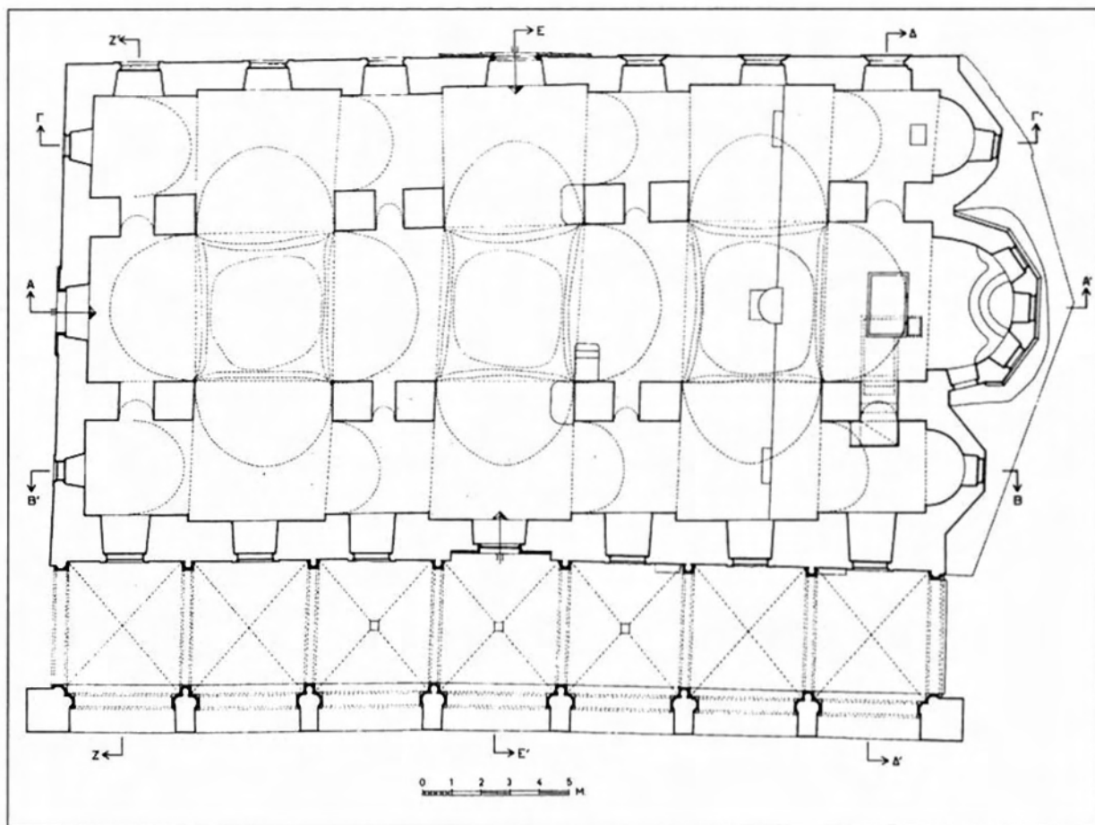
Σχ. 7. Κάτοψη.
