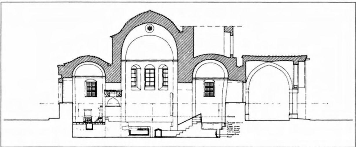
Σχ. 12. Τομή Δ-Δ'.
