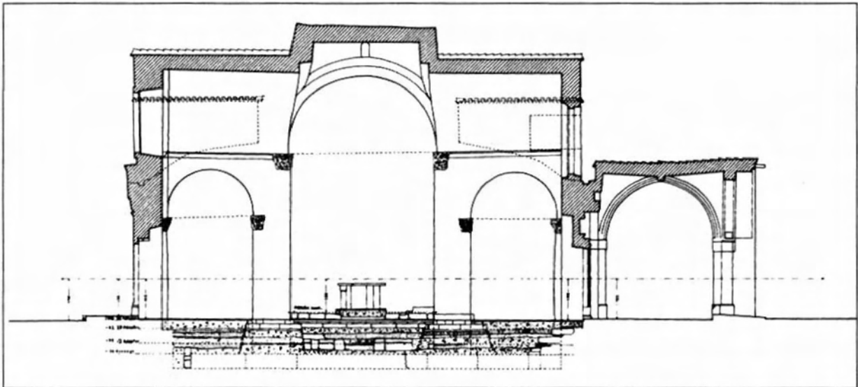
Σχ. 4. Τομή Ε-Ε'.
