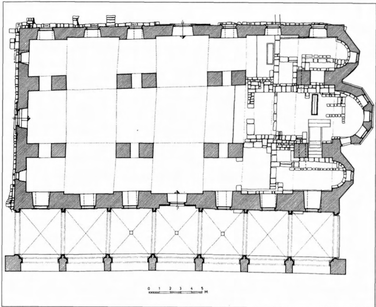
Σχ. 6. Κάτοψη.
