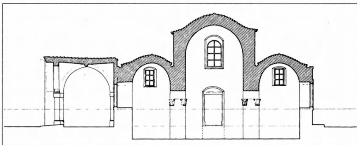
Σχ. 8. Τομή Z-Z.
