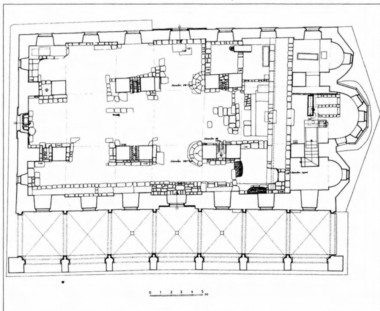
Σχ. 5. Κάτοψη.
