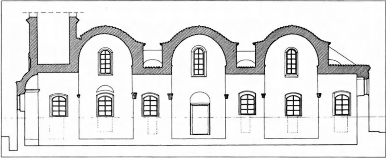
Σχ. 10. Τομή Β-Β'.
