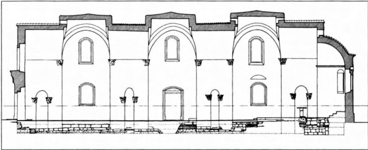
Σχ. 3. Τομή Α-Α'.
