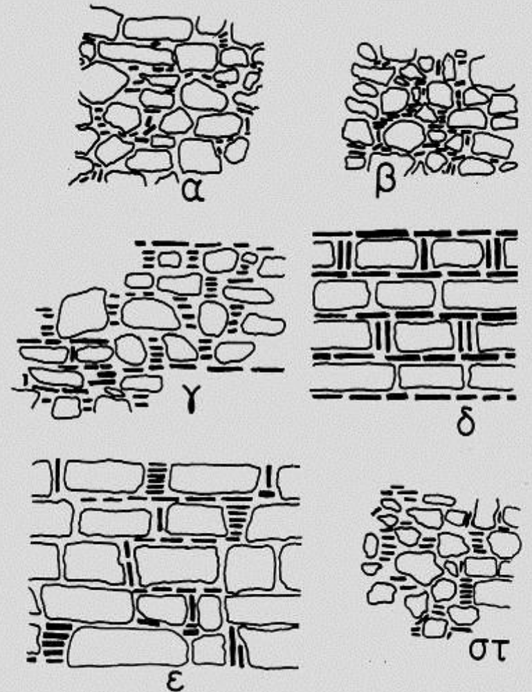
Σχ. 2. Κάστρο Ἰωαννίνων. Παραδείγματα τειχοδομιῶν: α, β = τείχος ὁδοῦ Ἰουστινιανοῦ (Τ1-Τ1'). γ = πύλη ἀκρόπολης Δημ. Μουσείου (ΠΛ1). δ, ε = πύργος τοῦ Θεωμᾶ (Π13). στ. = τείχος Τ3-Τ3'.
