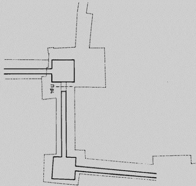
Σχ. 6. Κάτοψη δυτικού κόμβου. Πρώτη ρωμαϊκή φάση.
