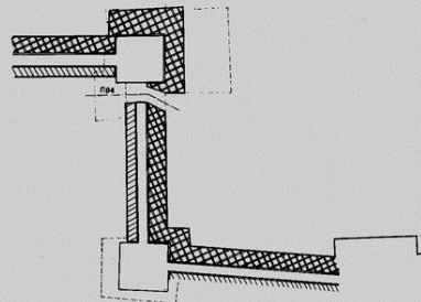
Σχ. 8. Κάτοψη δυτικού κόμβου. Δεύτερο τέταρτο 7ου αι. μ.Χ. (έργο Πύρρου).
