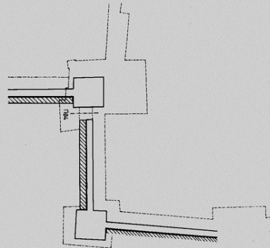
Σχ. 7. Κάτοψη δυτικού κόμβου. Φάση εποχής Ιουλιανού.
