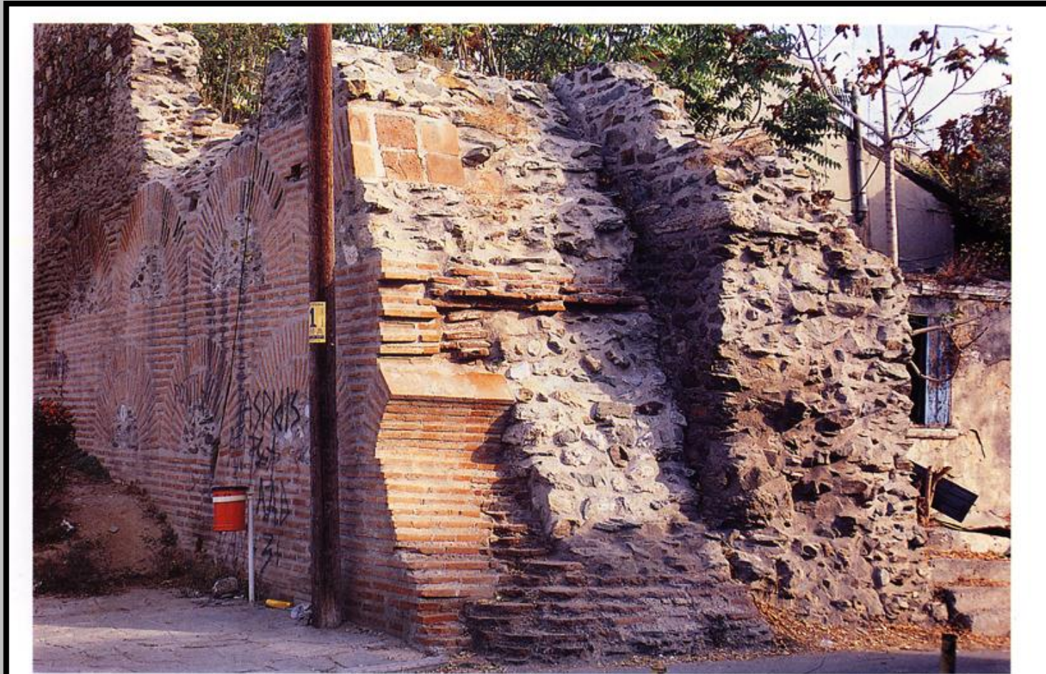
Εικ. 73. Ρήγμα του περιβόλου στην οδό Σαχτούρη. Εξωτερικά διακρίνεται η παλαιοχριστιανική οχύρωση μετά τις πρόσφατες επισκευές και εσωτερικά η ρωμαϊκή, σε επαφή.
