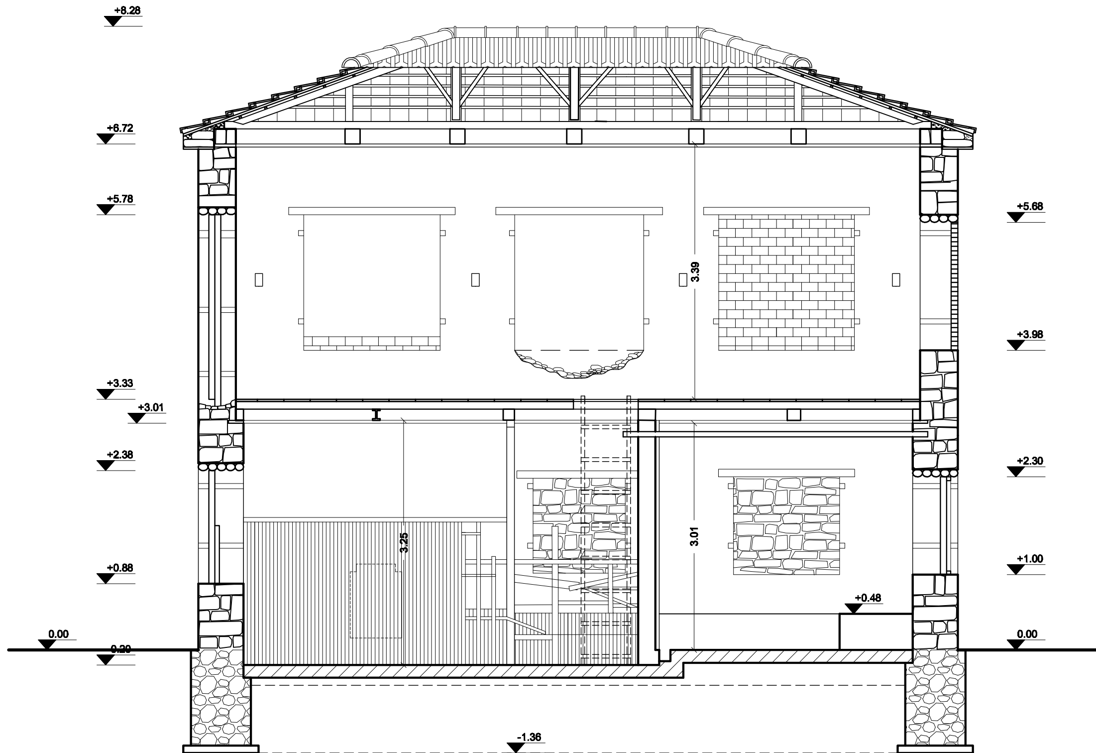
TOMH A-A' KAIMAKA 1:50
