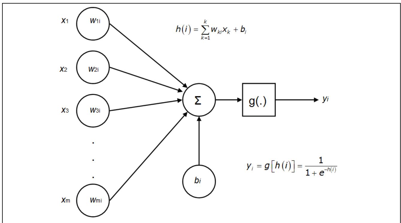
Εικόνα 7.5: Ένας νευρώνας που δέχεται είσοδο από n διαφορετικούς νευρώνες. Η τιμή κάθε νευρώνα εισόδου πολλαπλασιάζεται με το αντίστοιχο συναπτικό βάρος και αθροίζεται (μαζί με την τιμή του bias) πριν περάσει από τη συνάρτηση ενεργοποίησης η οποία θα δώσει το τελικό αποτέλεσμα. Στο συγκεκριμένο παράδειγμα η συνάρτηση ενεργοποίησης είναι η μη συμμετρική σιγμοειδής.
