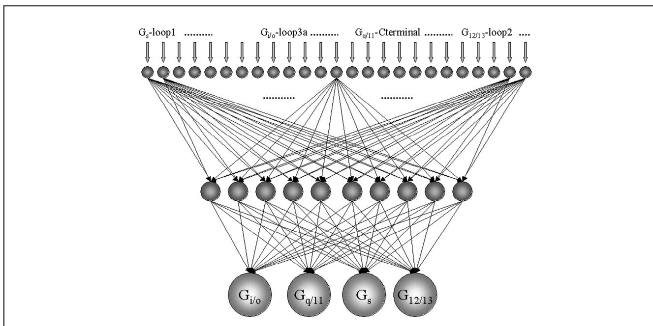
Εικόνα 7.27: Το νευρωνικό δίκτυο της μεθόδου PRED-COUPLE2. Σαν δεδομένα εισόδου χρησιμοποιούνται τα σκορ από τα rHMM που είχαν κατασκευαστεί με μια διαδικασία όμοια με το PRED-COUPLE.
