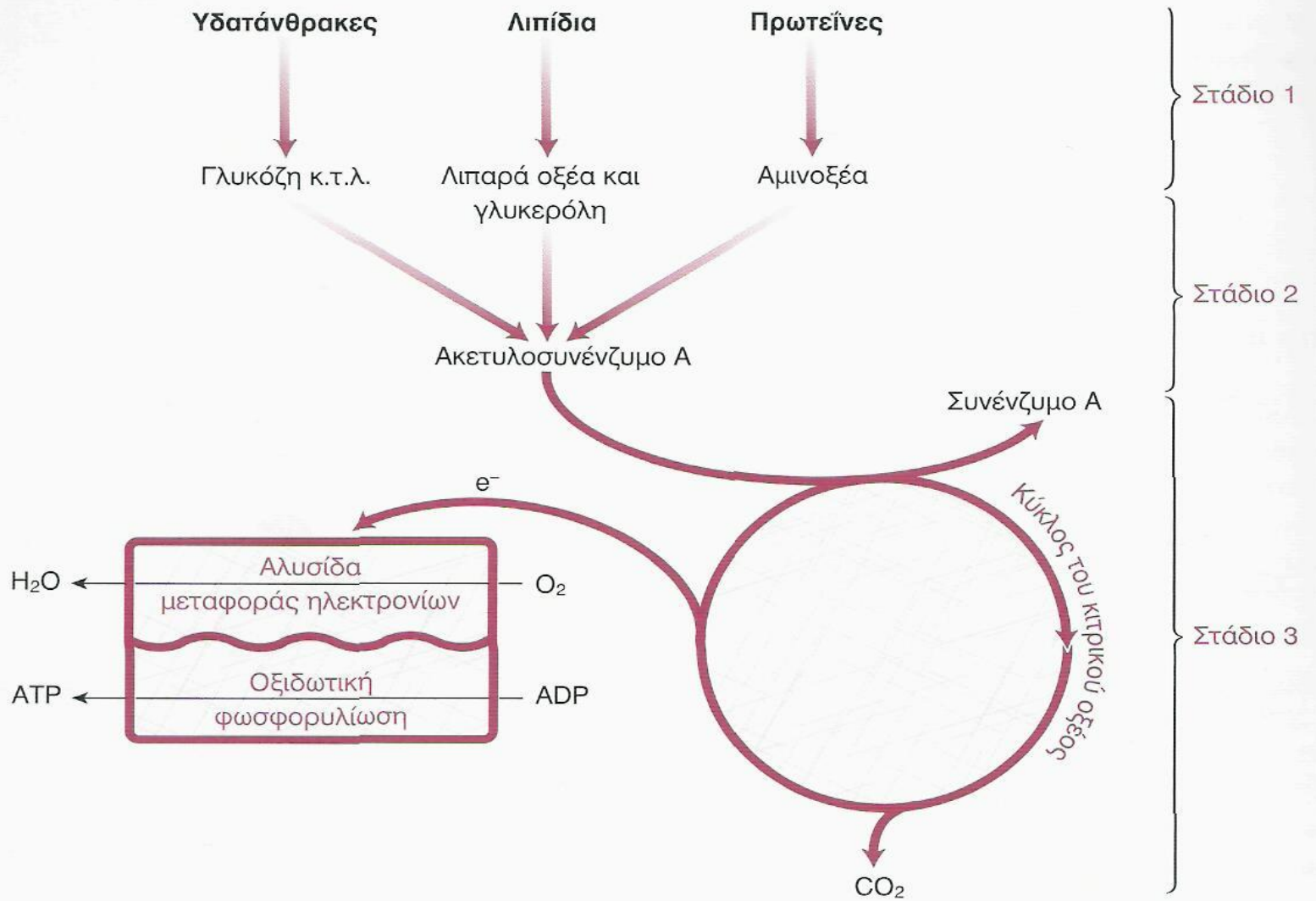
Εικόνα 2.10 Στάδια του καταβολισμού. Τα ζώα και οι άνθρωποι εξαγάουν ενέργεια από τα τρόφιμα σε τρία στάδια. Στο στάδιο 1, μεγάλα μόρια διασπώνται σε μικρότερα μόρια. Στο στάδιο 2, αυτά μετατρέπονται σε ακετυλοσυνένζυμο Α (με εξαίρεση ένα αριθμό αμινοξέων που ακολουθεί διαφορετική πορεία). Στο στάδιο 3, η ακετυλομάδα του ακετυλοσυνενζύμου Α διοχετεύεται στον κύκλο του κιτρικού οξέος –αφήνοντας το συνένζυμο Α πίσω– και μετατρέπεται σε διοξίδιο του άνθρακα. Τα ηλεκτρόνια που παράγονται στον κύκλο διοχετεύονται στην αλυσίδα μεταφοράς ηλεκτρονίων, και η ενέργεια που απελευθερώνεται τροφοδοτεί τη σύνθεση ATP μέσω της οξειδωτικής φωσφορυλίωσης.
