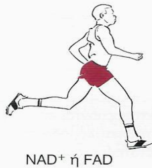
Εικόνα 2.9 Οξειδοαναγωγική σκυταλοδρομία. Οι μεταβολίτες οξειδώνονται παρέχοντας τα υδρογόνα τους σε ενδιάμεσα οξειδωτικά όπως τα \text{NAD}^+ και \text{FAD} . Τα \text{NADH} και \text{FADH}_2 που σχηματίζονται, δίνουν τα υδρογόνα στο οξυγόνο, το τελικό οξειδωτικό, και το μετατρέπουν σε νερό.
